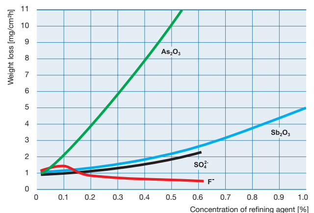
Material consumption due to refining agents (J. Vach and V. Süsser: Schmelzen von Gläsern in kleinen elektrischen Öfen, 46. Glastechnische Tagung, Wiesbaden, 1972)
